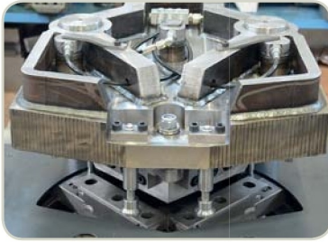
Açı Ayarlı Bıçaklar (Standart) Angle Adjustable Blades
